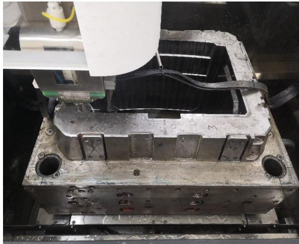
Cooler Die insert wirecut Machining
