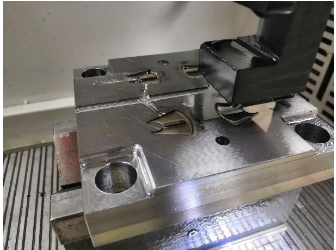
एसपीएम फिक्सचर पार्ट के लिए सीएनसी ईडीएम मशीनिंग
