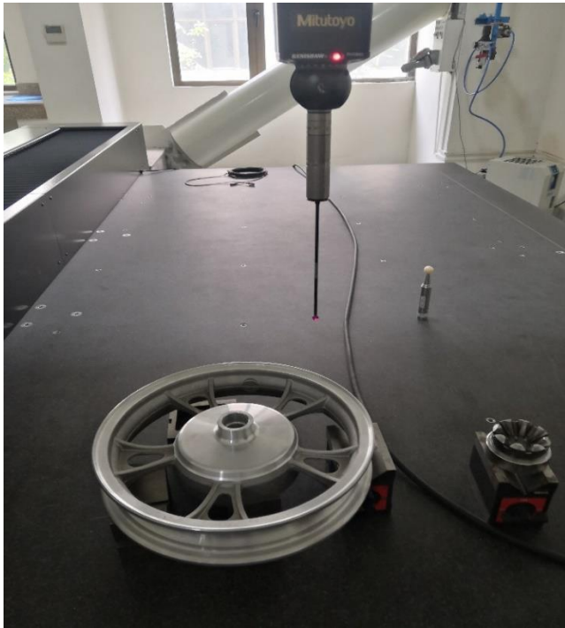
ईवी 2 व्हीलर अलॉय व्हील निरीक्षण
