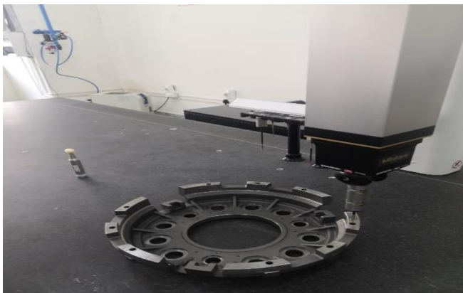
क्लच प्लेट इंस्पेक्शन
