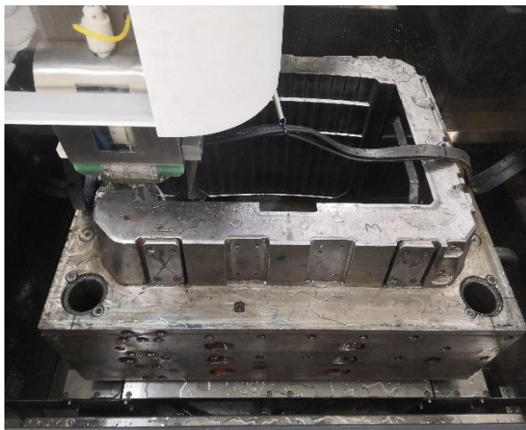
कूलर ड्राई इन्सर्ट वायरकट मशीनिंग
