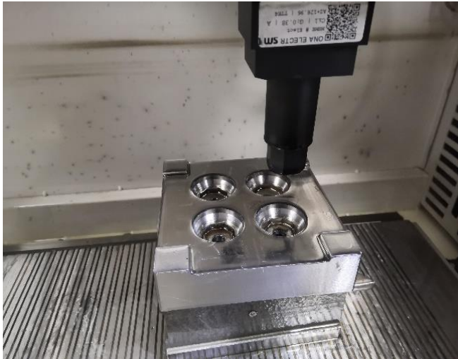
रबर मोल्ड प्रोफाइल के लिए सीएनसी ईडीएम मशीनिंग
