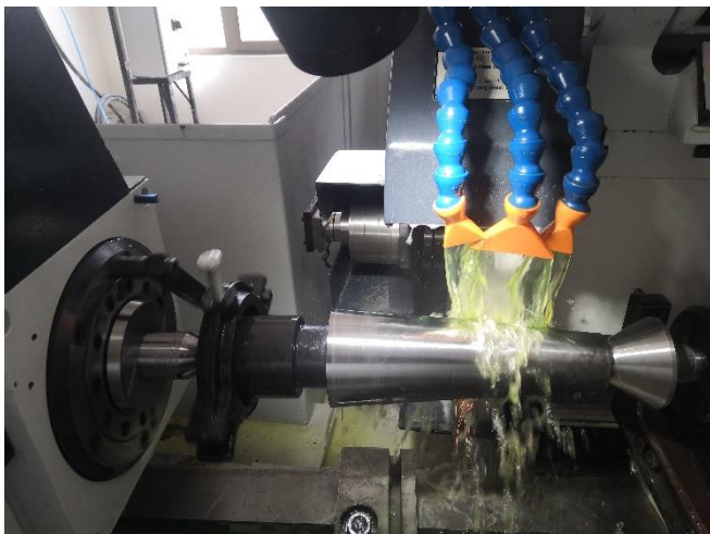
मैन्ड्रेल्स पर टेपर प्रोफाइल ग्राइंडिंग
