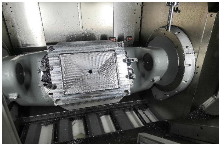
मोल्ड बेस पार्ट्स के लिए सीएनसी 5 एक्सिस मशीनिंग
